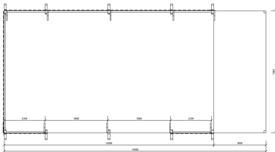
Figur 2: Plantegning
